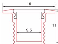
ΠΡΟΦΙΛ ΧΩΝΕΥΤΟ PROFILE RECESSED SINGLE
