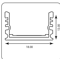
ΠΡΟΦΙΛ ΕΞΩΤΕΡΙΚΟ PROFILE EXTERNAL SINGLE
