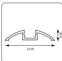
ΠΡΟΦΙΛ ΕΞΩΤΕΡΙΚΟ ΟΒΑΛ PROFILE EXTERNAL SINGLE OVAL
