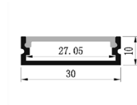
ΠΡΟΦΙΛ ΕΞΩΤΕΡΙΚΟ PROFILE EXTERNAL SINGLE
