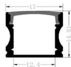
ΠΡΟΦΙΛ ΕΞΩΤΕΡΙΚΟ PROFILE EXTERNAL SINGLE
