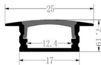
ΠΡΟΦΙΛ ΧΩΝΕΥΤΟ PROFILE RECESSED SINGLE
