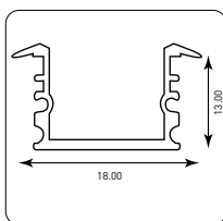
ΠΡΟΦΙΛ ΧΩΝΕΥΤΟ PROFILE RECESSED SINGLE
