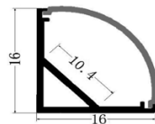
ΠΡΟΦΙΛ ΓΩΝΙΑ PROFILE SINGLE CORNER
