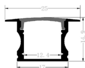
ΠΡΟΦΙΛ ΧΩΝΕΥΤΟ PROFILE RECESSED SINGLE
