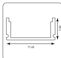
ΠΡΟΦΙΛ ΕΞΩΤΕΡΙΚΟ ΜΑΥΡΟ PROFILE EXTERNAL SINGLE BLACK
