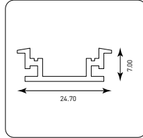
ΠΡΟΦΙΛ ΧΩΝΕΥΤΟ ΜΑΥΡΟ PROFILE RECESSED SINGLE BLACK
