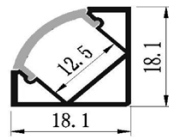
ΠΡΟΦΙΛ ΓΩΝΙΑ PROFILE SINGLE CORNER
