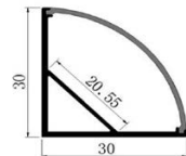
ΠΡΟΦΙΛ ΔΙΠΛΟ ΓΩΝΙΑ PROFILE DOUBLE
