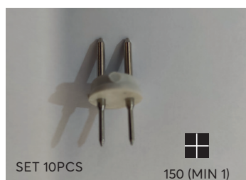
ΚΑΡΦΑΚΙ ΣΥΝΔΕΣΗΣ ΑΠΟ ΠΑΡΟΧΗ ΣΕ ΦΩΤΟΣΩΛΗΝΑ
